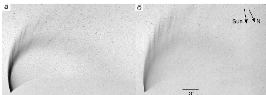
Рис. 3. Изображения кометы C/2006 P1 (Мак-Нота): а — модель, б — наблюдения 24 января 2007 г.
