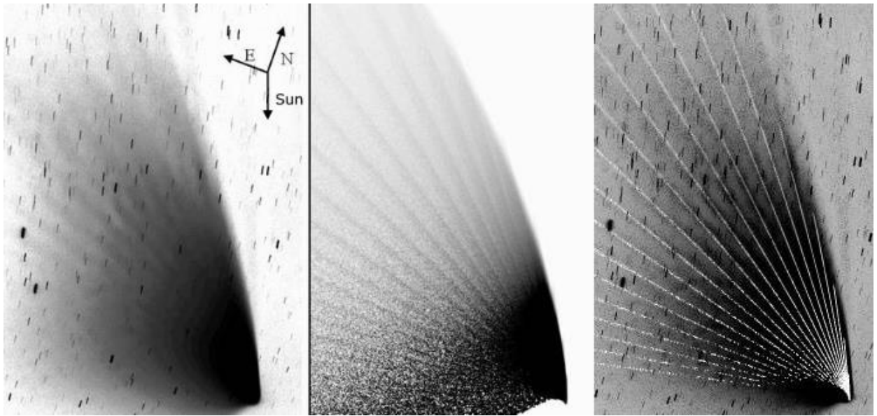
Рис. 3. Зліва направо розміщено спостережене зображення комети C/2011 L4 (PanSTARRS), модельне зображення і спостережене зображення зі стилізованим накладенням модельних смуг. Розмір зображень – 1.7^\circ \times 2.65^\circ .
