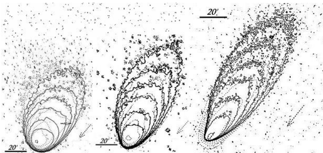
Рис. 1. Зіставлення ізофот комети C/1995 O1 (Hale–Bopp) для дат 8 лютого, 18 лютого і 7 березня 1997 року (зліва направо). Суцільні лінії – модельні, точкові лінії – спостережні ізофоти. Приведено масштаб і напрямок на Сонце (стрілкою).
