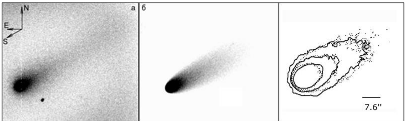
Рис. 4. Зліва направо розміщено спостережене та модельне зображення комети C/2012 S1 (ISON), а також модельні (точкові) й спостережені (суцільні) ізофоти. Зазначено напрямки на Сонце, північ, схід, а також бар 10000 \text{ км} = 7.6'' .
