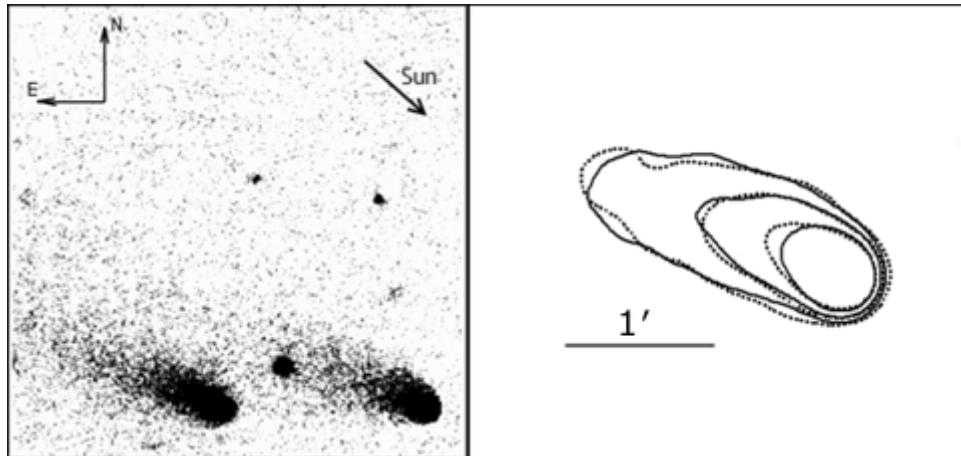
Рис. 5. Зліва направо розміщено спостережене та модельне зображення комети C/2012 K5 (LINEAR), а також модельні (суцільні) й спостережні (точкові) ізофоти. Зазначено напрямки на Сонце, північ, схід, а також масштаб.
